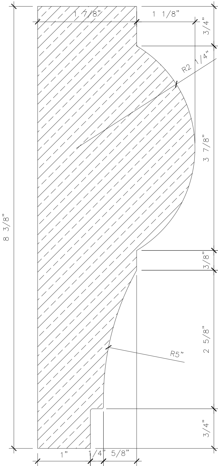
1 PROFILE 203-M
