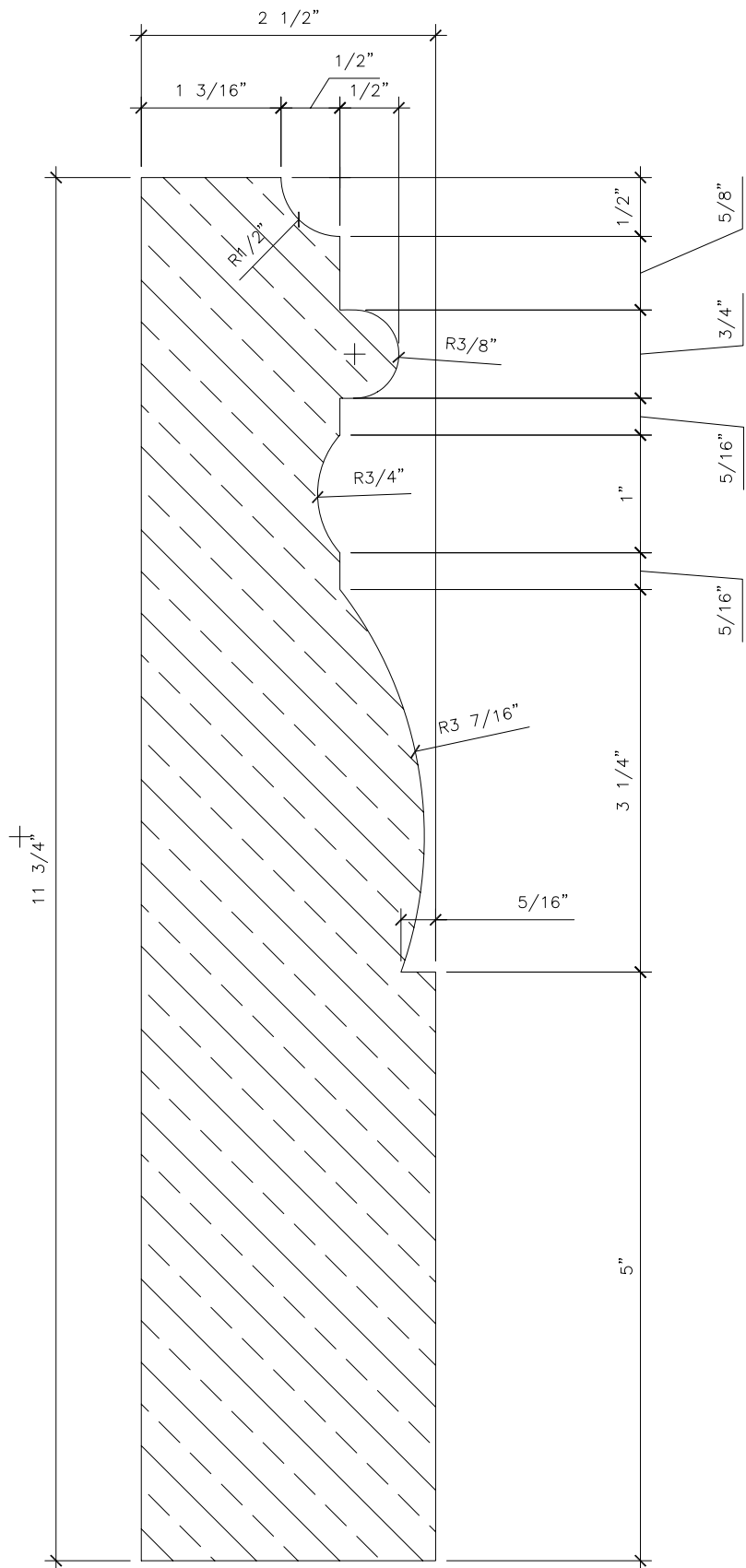
1 PROFILE 901-M
