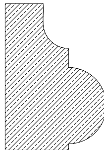
PROFILE 401-T 17 LBS. PER LINEAR FOOT
