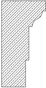
PROFILE 201-I 12 LBS. PER LINEAR FOOT
